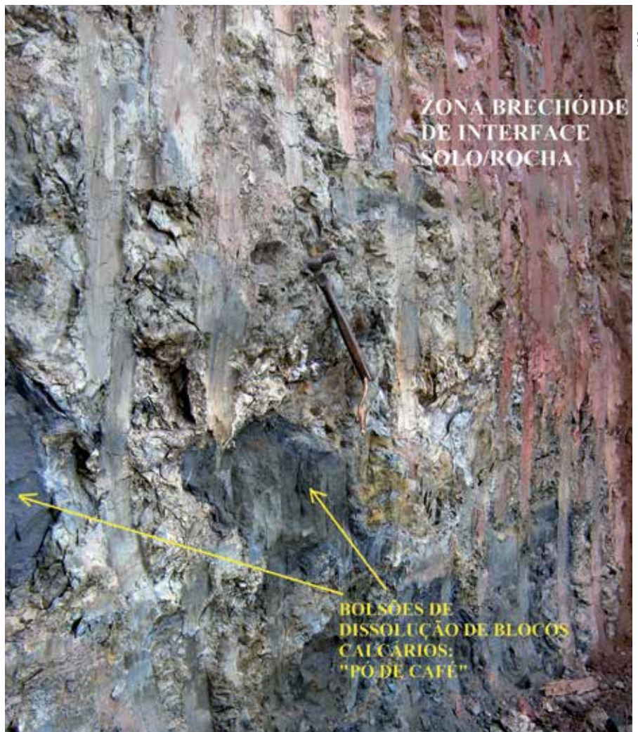
Figura 9 – Terraplenagem que expôs porção da zona brechoide da interface solo/rocha permitindo sua investigação detalhada. Notar convivência espacial de materiais argilosos claros e avermelhados e bolsões com material pulverulento ("pó de café") originário da dissolução de núcleos calcários
