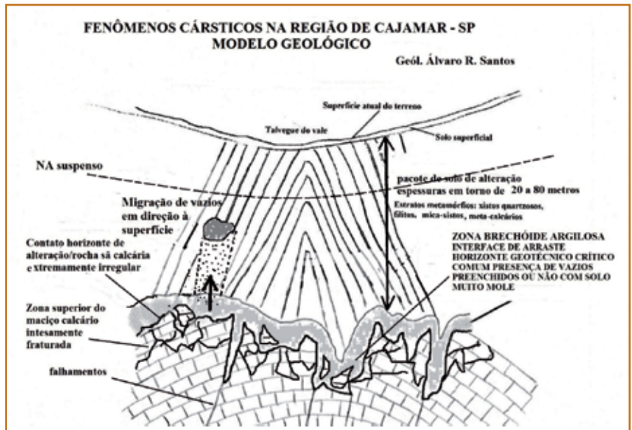
Figura 8 – Croqui do novo modelo geológico para os fenômenos cársticos da região de Cajamar –SP
