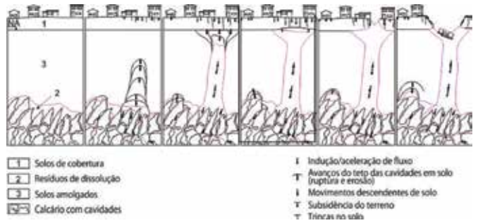
Figura 3 – O modelo originalmente proposto pelo IPT, indicando um processo de migração de solo para os vazios em rocha e a migração do vazio formado em direção à superfície
