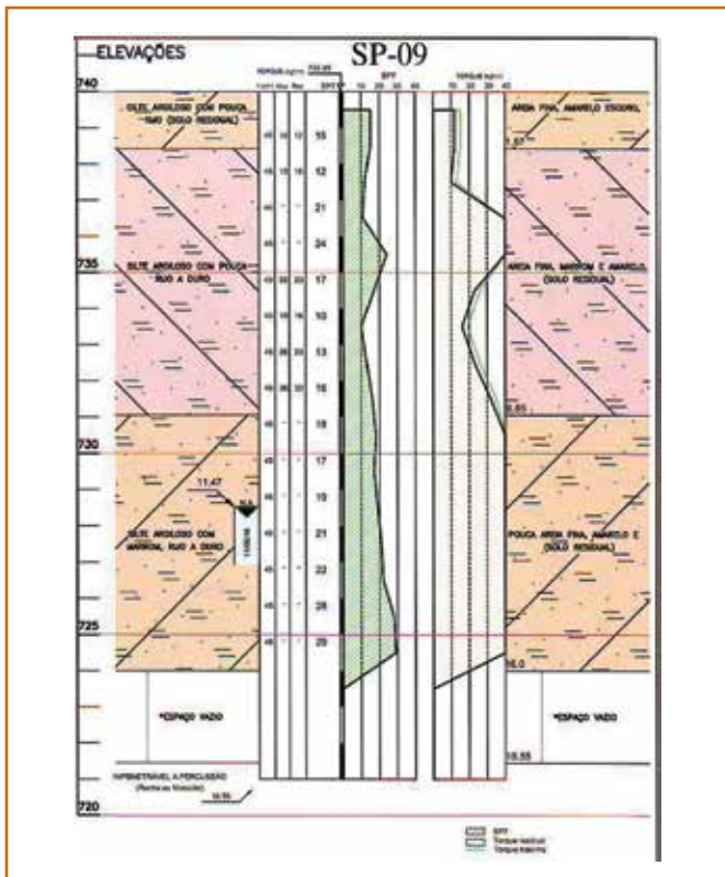
Figura 4 – Perfil típico de sondagem a percussão em terrenos cársticos da região de Cajamar. Imediatamente acima do topo rochoso aparecem bolsões totalmente vazios ou preenchidos de solo muito mole
